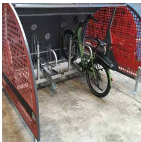
Supports de stationnement intégrés numérotés avec arceaux pour 5 vélos
